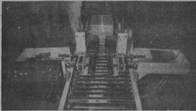
Máquina automática codificadora diseñada por investigadores y alumnos de la Facultad de Ingeniería, para la industria alimentaria.
