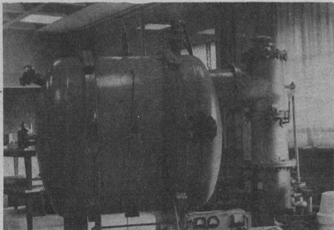
Cámara de Blancos en donde se lleva a cabo la implantación de iones en muestras sólidas.
